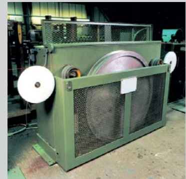
VB 40 Capstan
